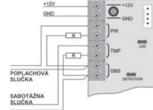
Príklad zapojenia detektora JS-20 LARGO do jednoducho vyváženej slučky pre ústredne JA-63 a JA-65 (svorky GBS sú použité ako pomocné).
